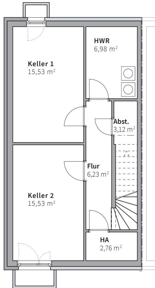
Untergeschoss
