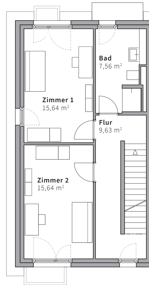
Obergeschoss
