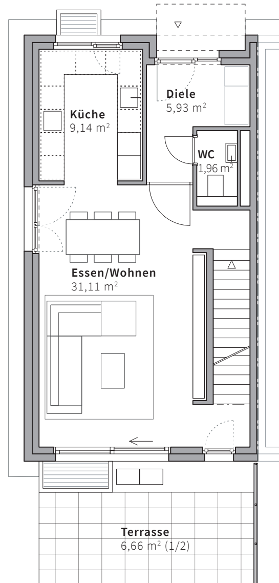
Erdgeschoss
