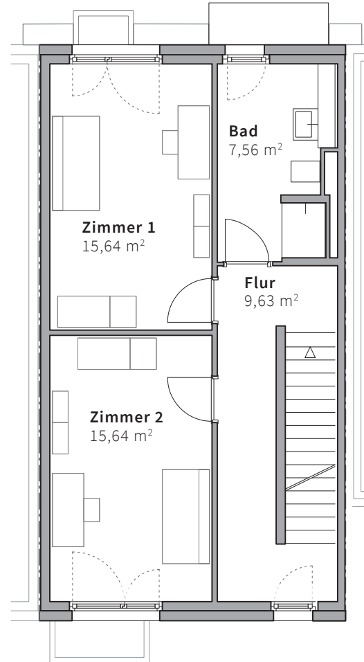
Obergeschoss
