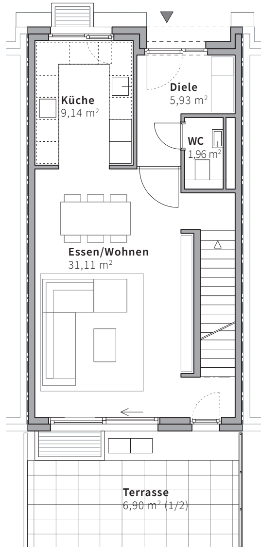
Erdgeschoss
