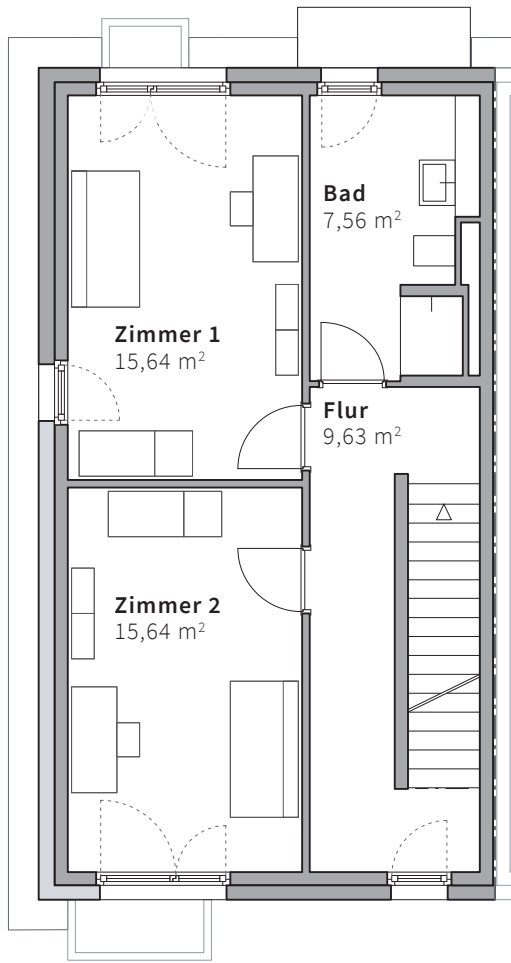
Obergeschoss
