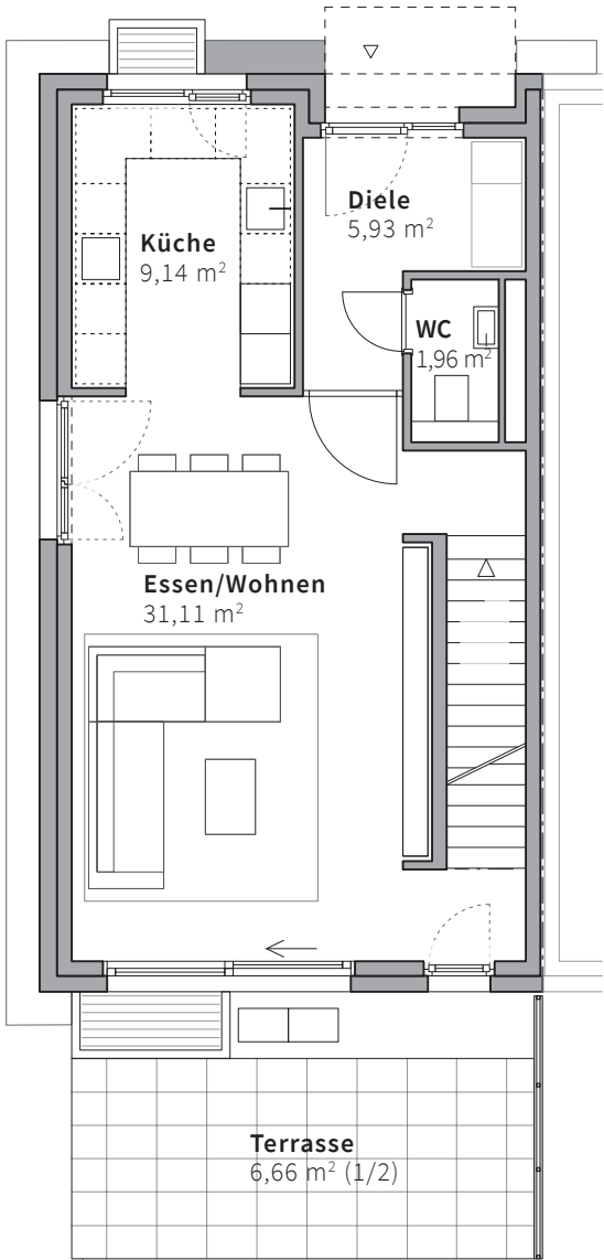
Erdgeschoss
