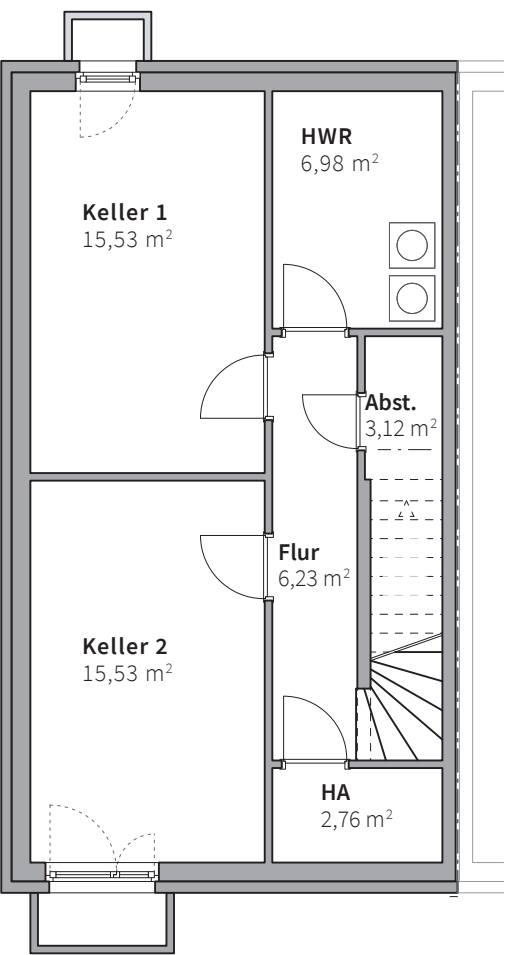
Untergeschoss
