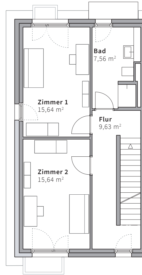
Obergeschoss
