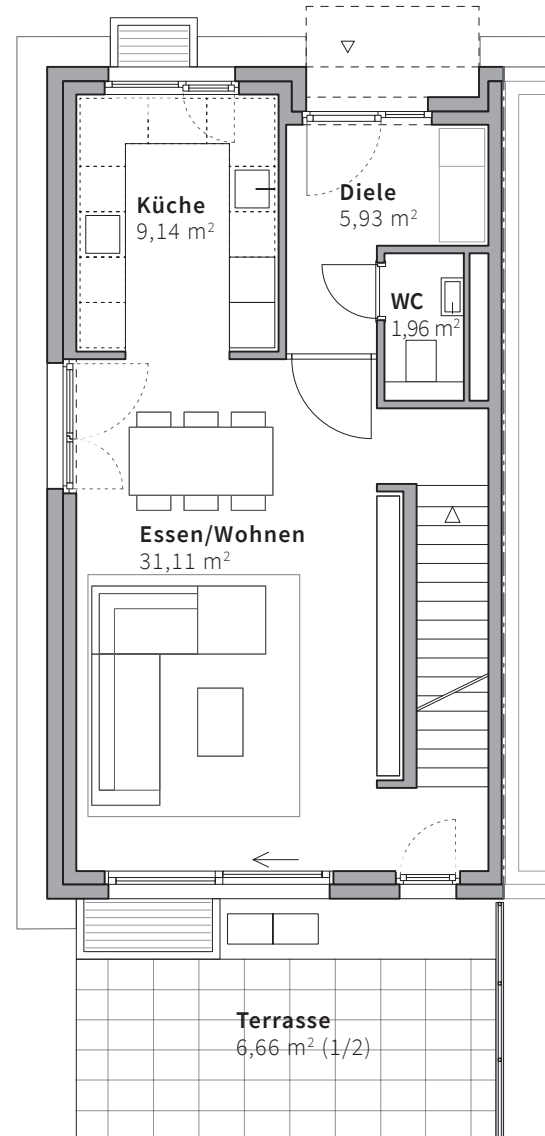
Erdgeschoss
